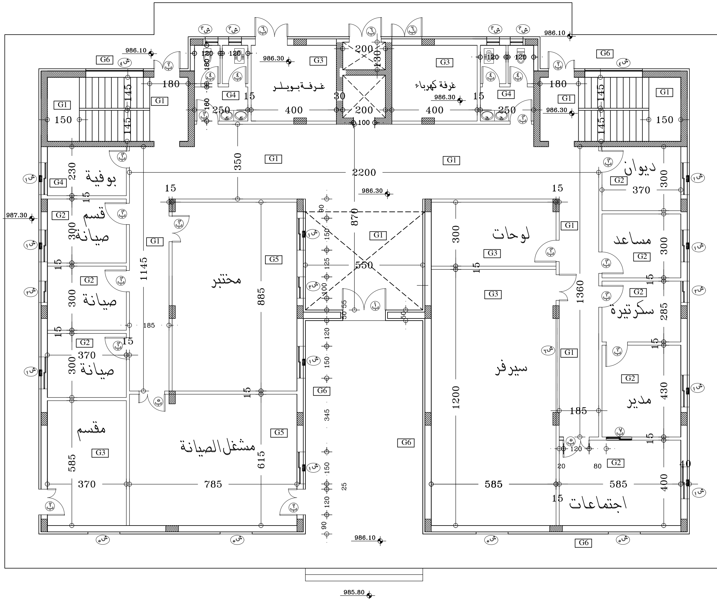
مخطط الطابق الارضي
